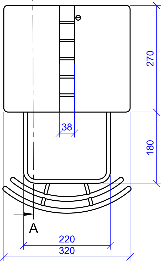
VISTA SUPERIOR
